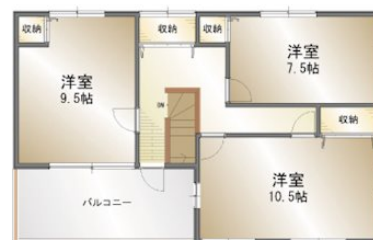
【2階間取り図】
