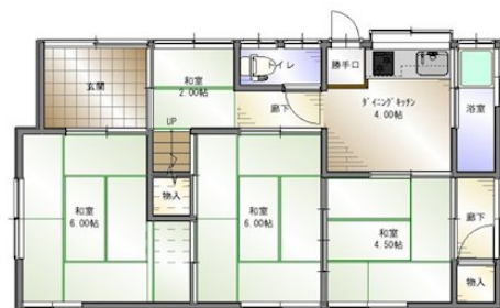
【1階 間取り図】
